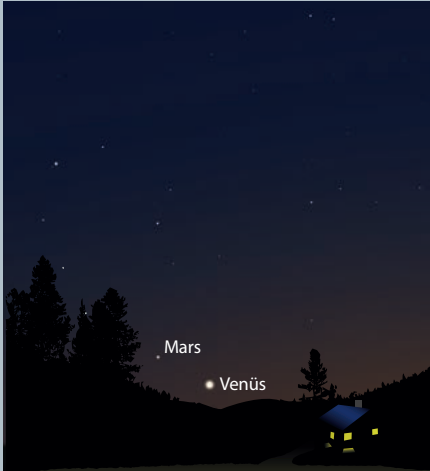
5 Temmuz günbatımı sonrası batı ufku
