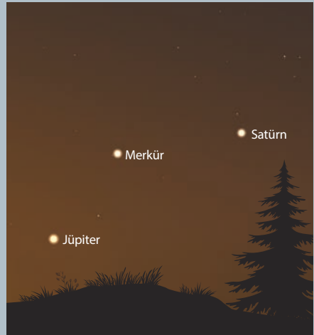
26 Şubat gün doğumundan önce doğu ufku
