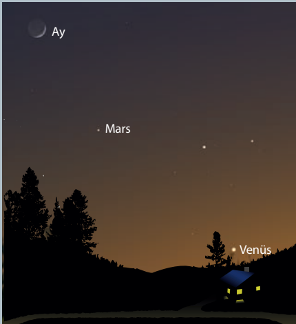
14 Haziran günbatımı sonrası batı ufku
