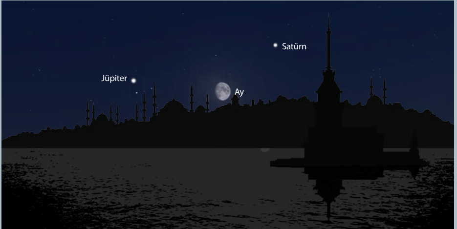
17 Eylül günbatımı sonrası güneydoğu ufku
