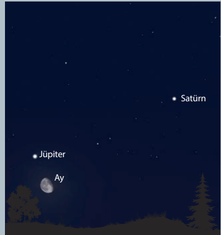
28 Haziran gece ortası güneydoğu ufku
