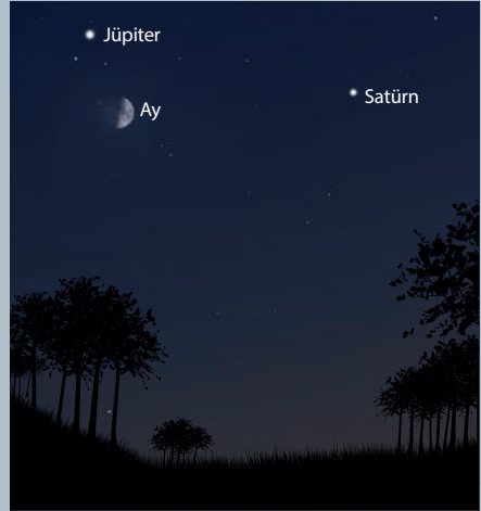
11 Kasım günbatımı sonrası güney yönü
