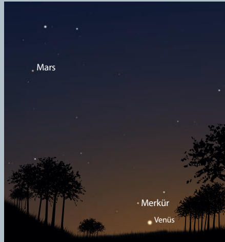
25 Mayıs günbatımı sonrası batı ufku
