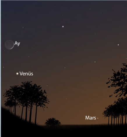
11 Ağustos günbatımı sonrası batı ufku
