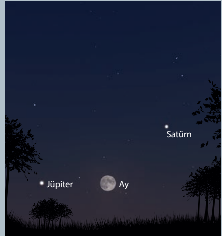
21 Ağustos günbatımı sonrası güneydoğu ufku
